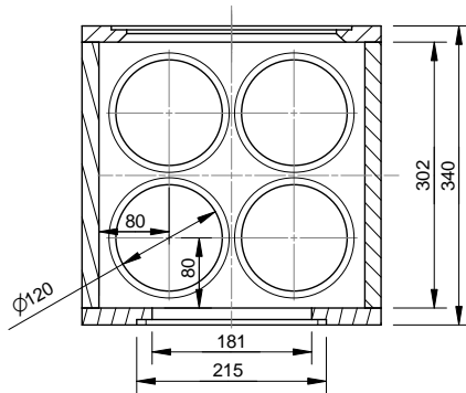
Schnitt B-B
